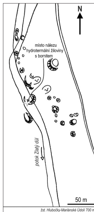
Obr. 1: Plánek stop po těžbě polymetalických rud na historickém ložisku Zlatý důl s vyznačením místa nálezu hydrotermální žiloviny s bornitem (kreslil J. Klomínský in Losert 1962, upraveno). Fig. 1: Plan of the tracks after mining of the polymetallic ore at the historical deposit Zlatý důl with the location, where the sample of bornite-bearing vein was found (sketched by J. Klomínský in Losert 1962, modified).
