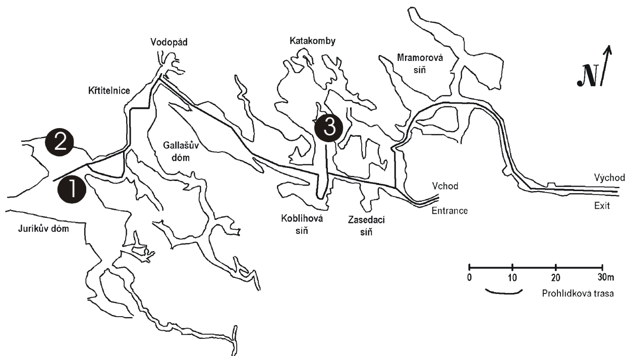
Obr. 1 – Schématická mapa Zbrašovských aragonitových jeskyní s vyznačenými lokalitami mikrobiologického vzorkování. 1 – Jurikův dóm – Opona, 2 – Jurikův dóm – Tunel, 3 – Koblihová síň.
