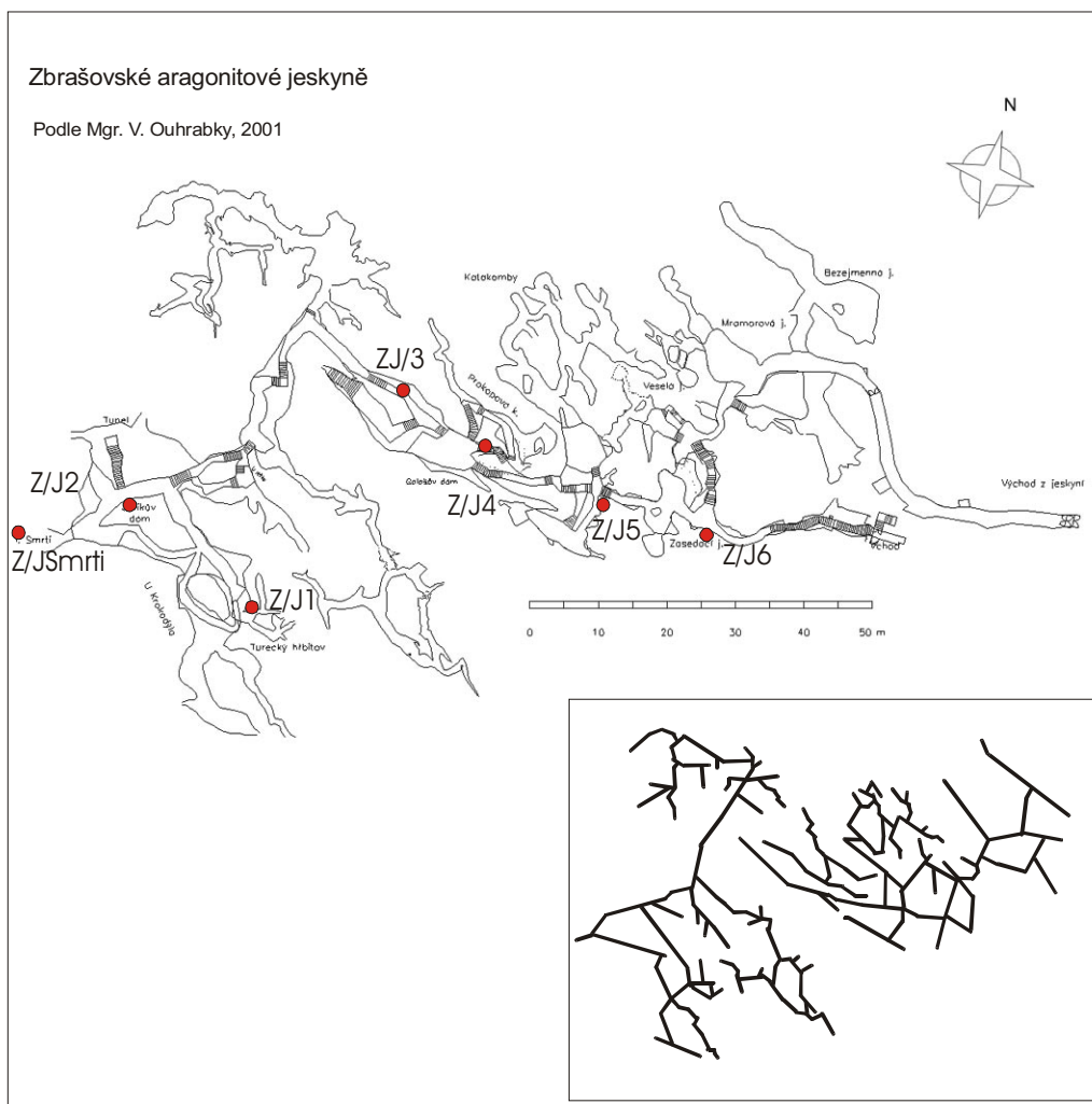
Obr. 1 – Schematický náčrt síťového modelu orientace krasových chodeb Zbrašovských jeskyní a lokalizace vzorků na konodonty.
