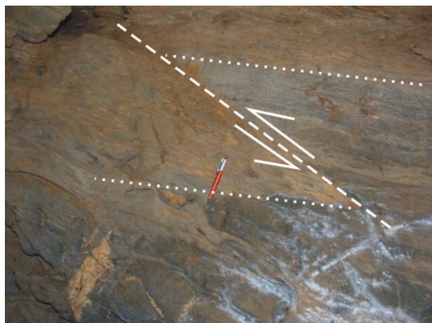
Obr. 4 – Doklad šupinové stavby vápenců – drobný přesmyk dislokující litologické rozhraní hlízatých a krinoidových organodetrinitických vápenců (směr pohybu generálně k JV).
