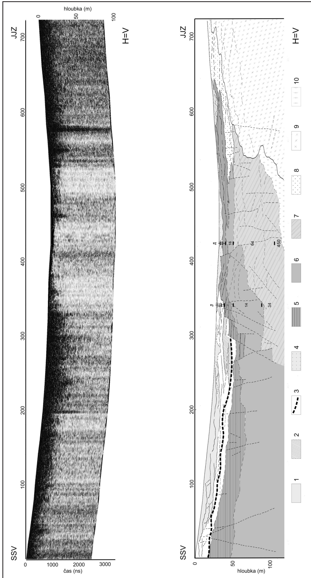
Obr. 1: Geofyzikální profil P0 přes nestabilní svah na novém sídlišti Brno-Medlánky, vrt Medlánky-1 je situován v místě nestabilního tělesa a), b) interpretace. Vysvětlivky: 1. vymezení stávajícího sesuvu, 2. vymezení staršího sesuvu, 3. báze sesuvných pohybů, 4. kvartér, 5. jíly (nízké odpory, baden), 6. písčité jíly (baden), 7. písky (vyšší odpory, baden), 8. deluviální komplex, 9. skalní podloží (metabazit), 10.) zvětraliny a svahoviny (předbadenské).
