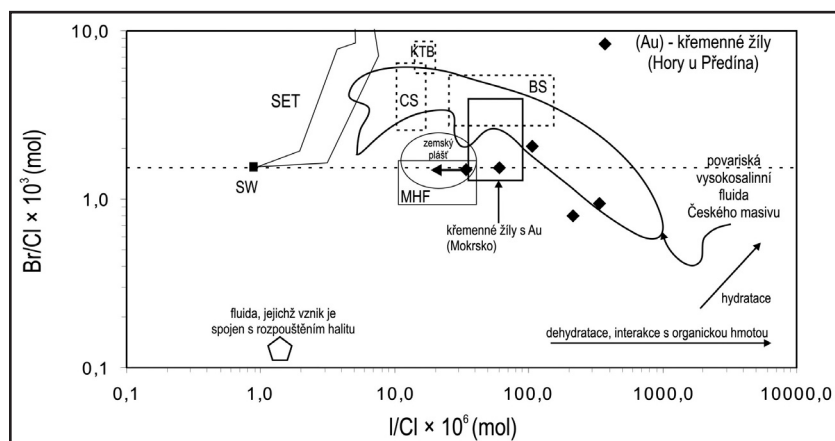
Obr. 2: Diagram I/Cl vs. Br/Cl vyluhů fluidních inkluzí z Hor u Předína a jejich srovnání s fluidy různého původu (upraveno podle Dolníčka et al. 2009, data pro Mokrsko převzata z Boiron et al. 2001). SW mořská voda, SET linie evaporace mořské vody, MHF nekontaminovaná magmatická hydrotermální fluida, CS solanky z kanadského štítu, BS solanky z baltického štítu, KTB hlubinné solanky navrtnané vrtem KTB (Bavorsko). ←♦ šipka značí směr skutečného umístění daného bodu (jód pod mezí stanovitelnosti).
